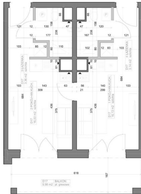
SCHEMAT BUDYNKU
