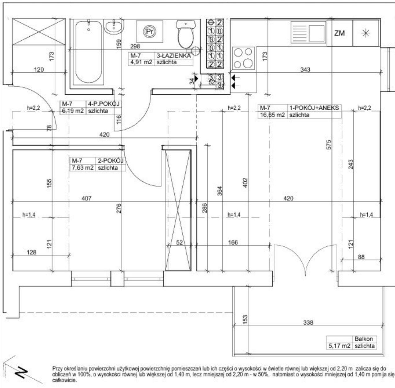
RZUT PODDASZA 1:500
