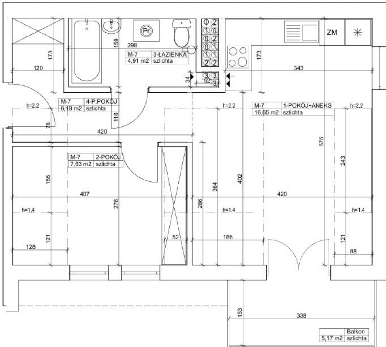
RZUT PODDASZA 1:500
