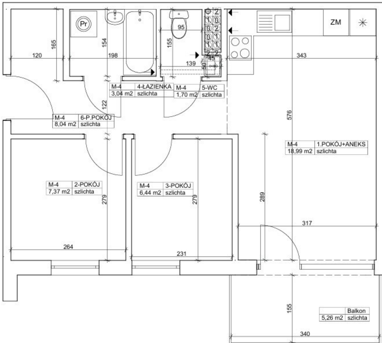
RZUT 2 PIĘTRA 1:500
