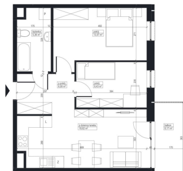
RZUT 1 PIĘTRA
